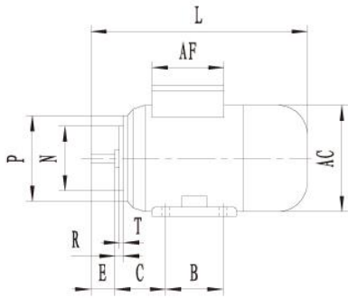
IM B34
