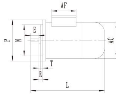
IM B5
