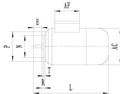
IM B14
