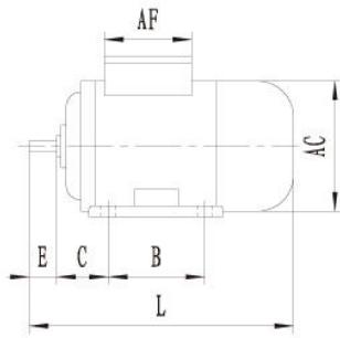
IM B3
