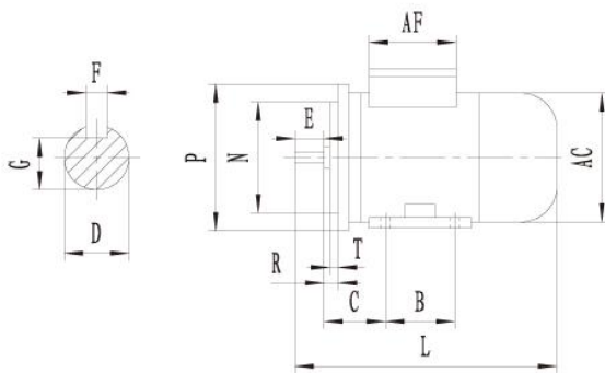
IM B35
